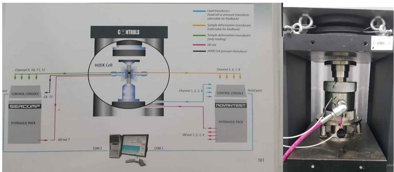
Hình 3. Sơ đồ kết nối hệ thống thí nghiệm và mẫu trong buồng nén sau khi lắp đặt
